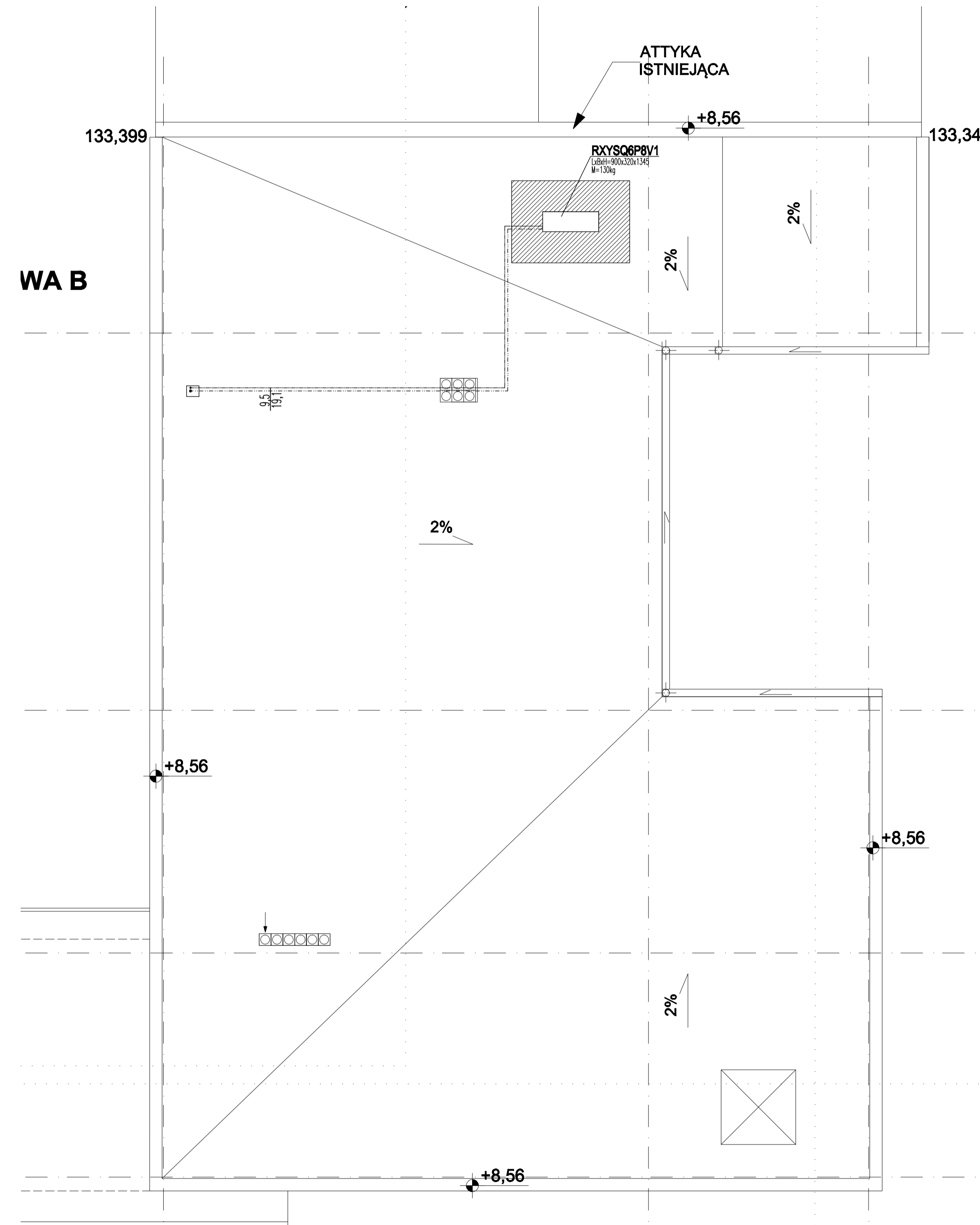
RZUT PODDASZA
